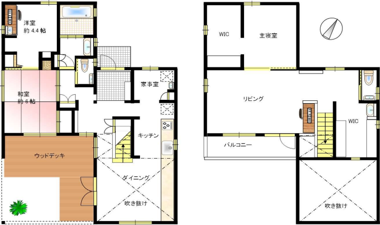
1F 2F 【概略図により現況を優先します】
